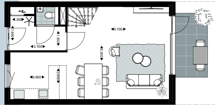
Begane grond
