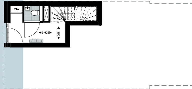
Begane grond
