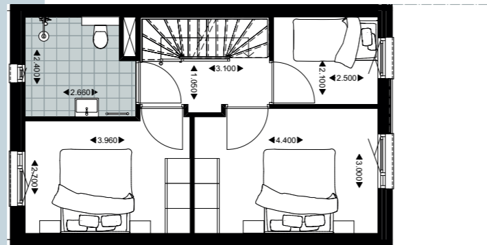
Eerste verdieping
