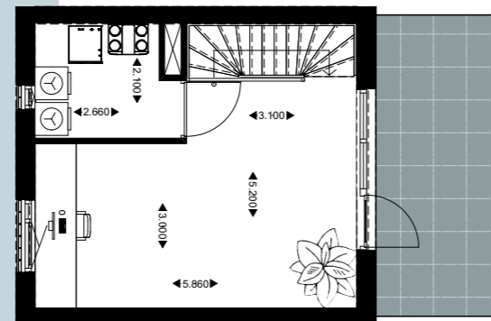
Tweede verdieping
