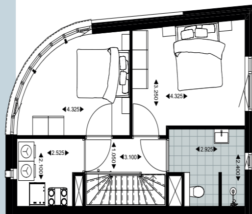
Tweede verdieping
