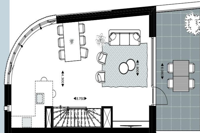
Eerste verdieping
